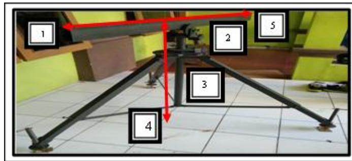
Gambar 2.2. Spesifikasi Perancangan Mekanik Peluncuran Roket
