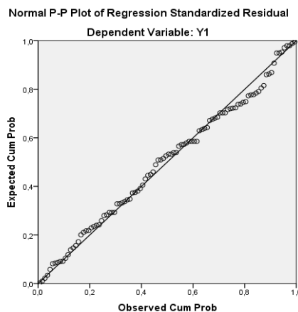
Gambar 2. Hasil Normalitas Data dengan Normal Probability Plots
