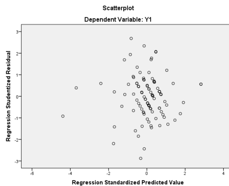
Gambar 1. Hasil Heterokedastisitas dengan Scatter Plot
