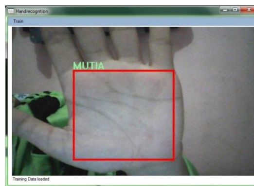
Gambar 3.3 Pengetesan database
