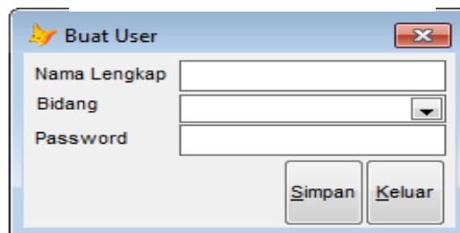
Gambar 4: Buat User
