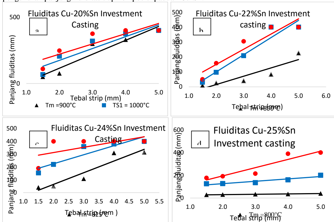
Gambar 3. Grafik panjang fluiditas (a) 20%Sn (b) 22%Sn (c) 24%Sn (d) 25%Sn
