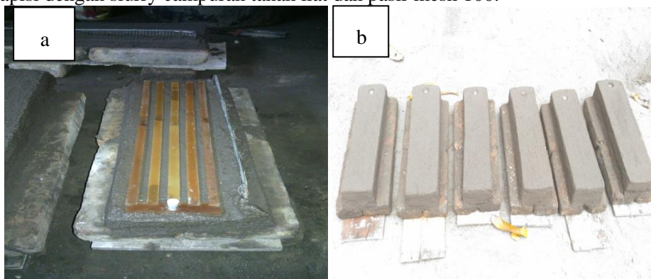
Gambar 4. Cetakan uji fluiditas (a) pola lilin (b) cetakan sudah dilapisi slurry
