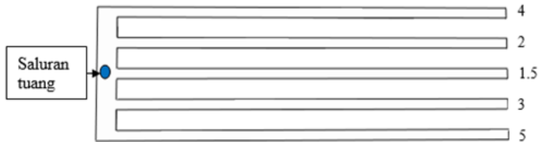
Gambar 3. Model dan dimensi cetakan uji fluiditas
