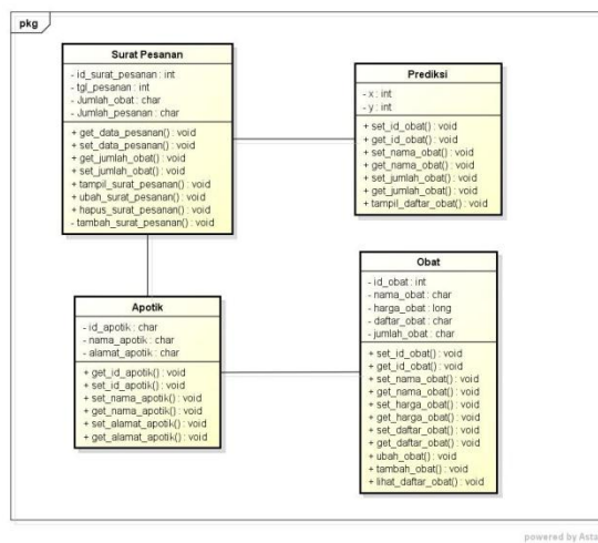
Gambar 4. Class Diagram Sistem Prediksi Kebutuhan Obat
