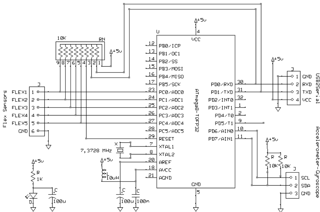
Gambar 6. Desain Skema Rangkaian
