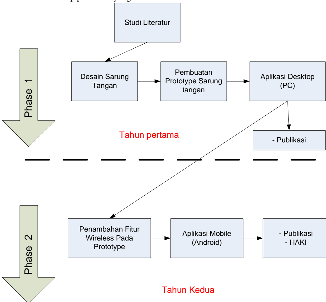
Gambar 5. Tahap penelitian
