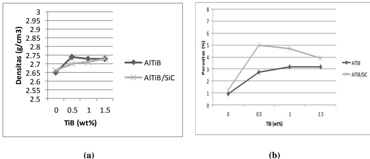
Gambar 1. Grafik (a) densitas AlTiB dan AlTiB/SiC, (b) tingkat porositas AlTiB dan AlTiB/SiC
