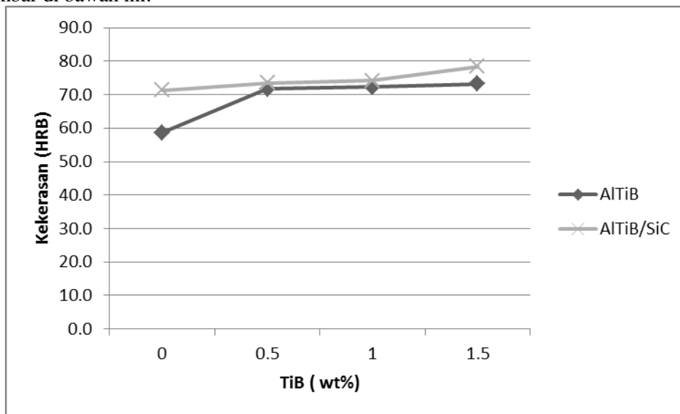
Gambar 2. Grafik kekerasan
