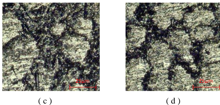
Gambar 3. Foto mikro matrik dengan variasi TiB ( a ) 0%, ( b ) 0,5%, ( c ) 1%, ( d ) 1,5%.
