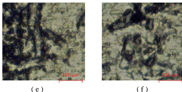
Gambar 4. Foto mikro ( e ) matrik AlSiMgTiB, ( f ) komposit AlSiMgTiB+SiC 5%.
