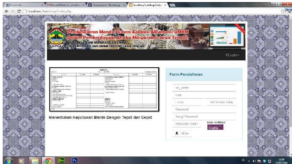
Gambar 5. Pendaftaran UMKM
