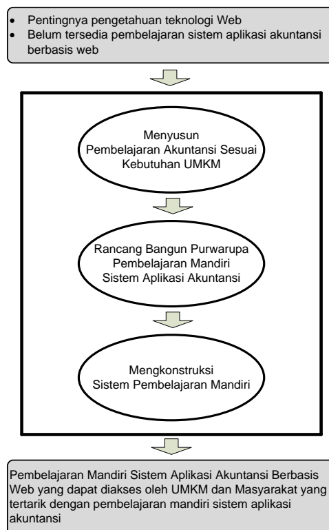
Gambar 3. Kerangka Pemikiran
