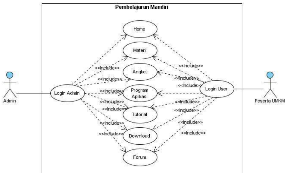
Gambar 4. Diagram Use Case untuk Pembelajaran
