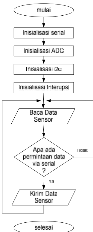
Gambar 5. Diagram Alir Program Mikrokontroler
