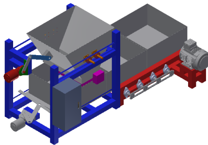
Gambar 2. Mesin pengisian curah tembakau
