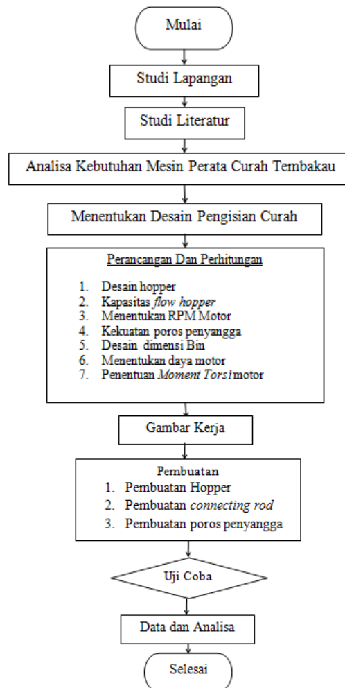
Gambar 1. Diagram alir perancangan sistem pengisian curah tembakau
