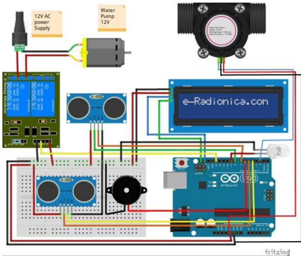
Gambar 1. Perancangan Wiring
