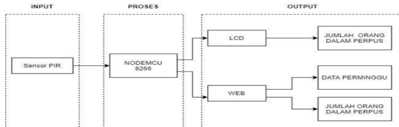
Gambar 1. Blok Diagram Sistem
