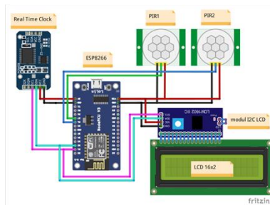
Gambar 2. Rangkaian Secara Keseluruhan
