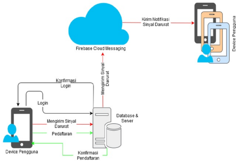
Gambar 5. Arsitektur Sistem
