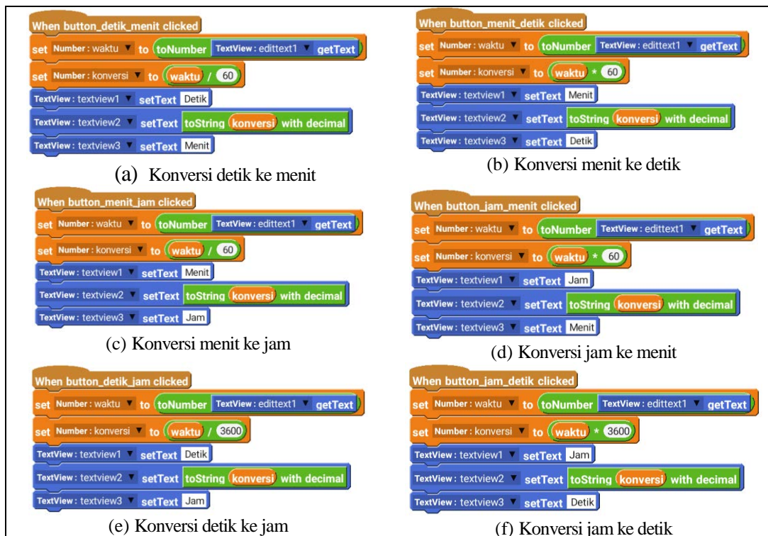
Gambar 8. Tampilan Logic Pada WaktuActivity.java
