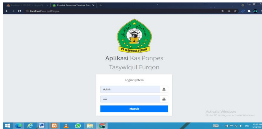
Gambar 6. Halaman Login
