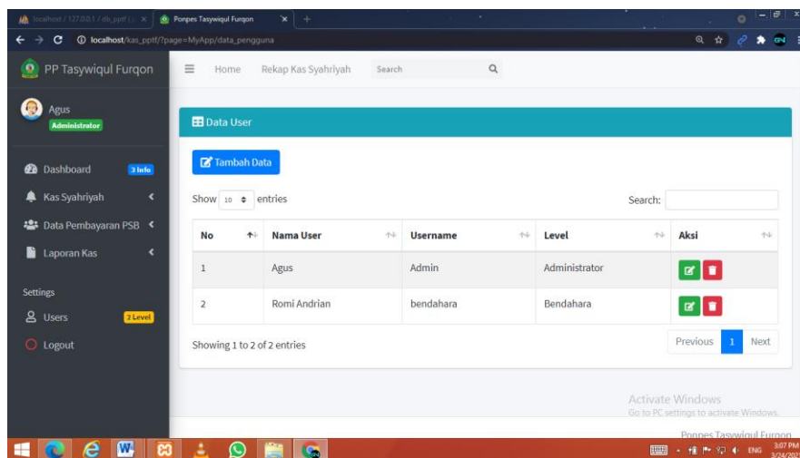
Gambar 13. Data Pengguna
