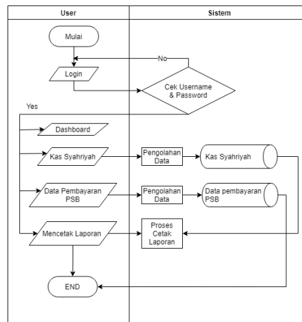
Gambar 1. Alur Sistem [5]
